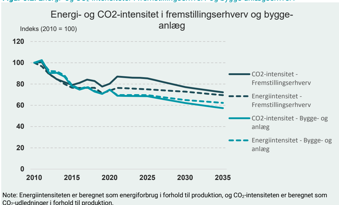
Figur 6.2: Energi- og CO 2 -intensiteter i fremstillingserhverv og bygge-anlæg
